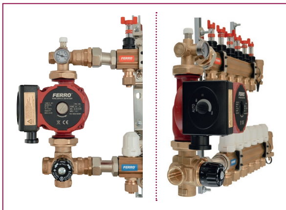
montaż GM z mimośrodami
